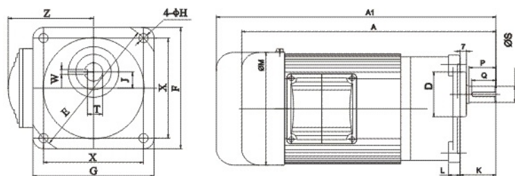
CV18外形图
