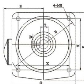
CV22-50外形图
